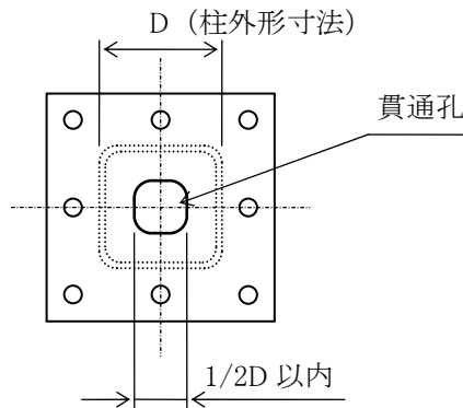
付図-1 ベースプレートの貫通孔
