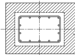
許容最大柱型寸法を超える場合の柱型拡大部の別途配筋領域
