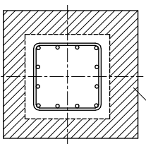
許容最大柱型寸法を超える場合の柱型拡大部の別途配筋領域
